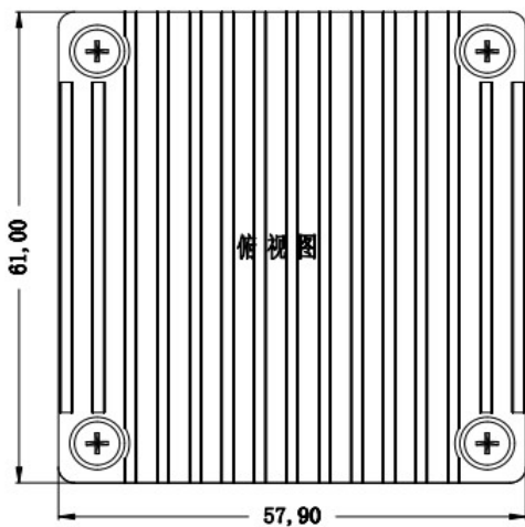
标准型+散热器 61*57.9*29.0mm
